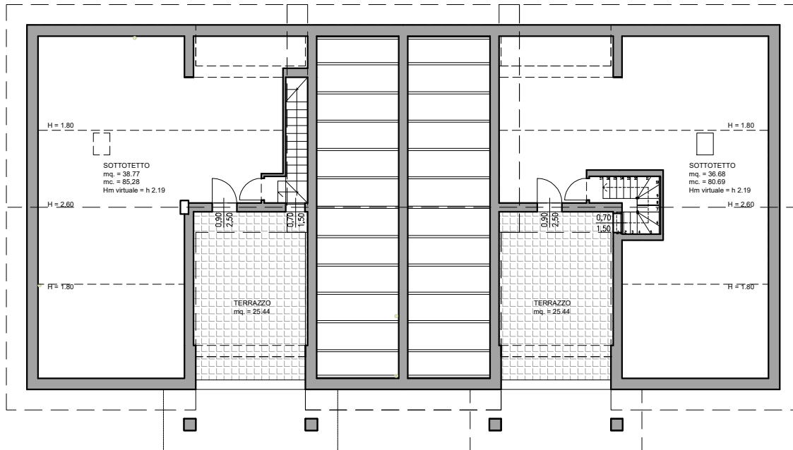
PIANO SOTTOTETTO
